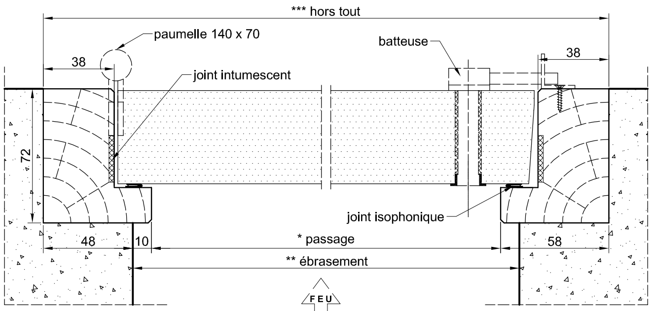
Coupe de principe
