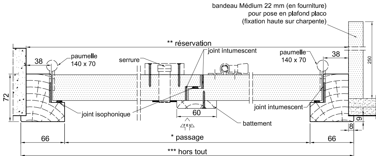
Coupe de principe
