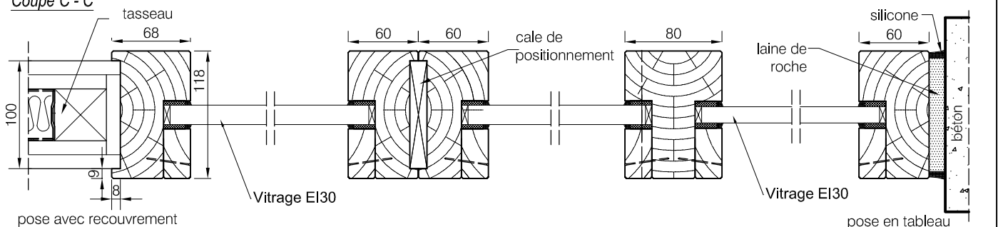
Coupe C - C
